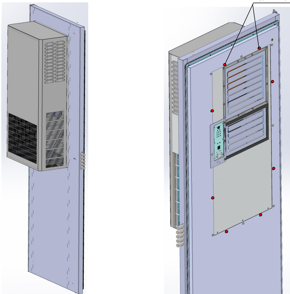
Рисунок 2 – Демонтаж блока кондиционера с двери
