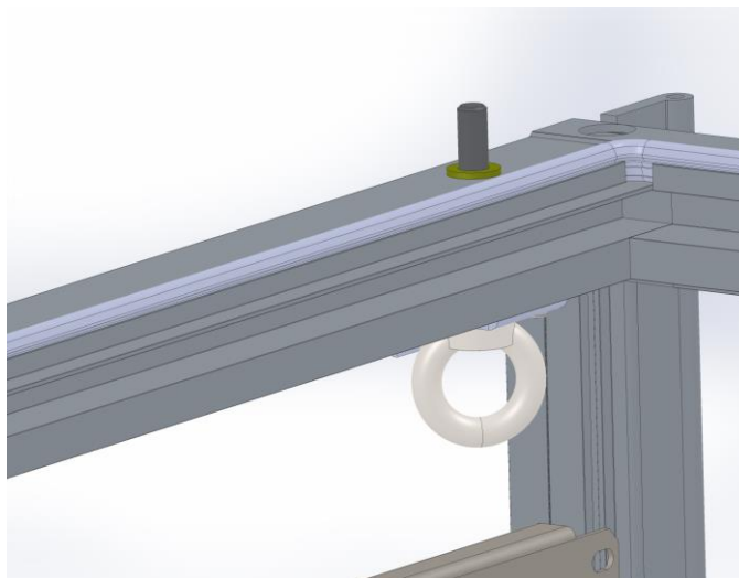
Рисунок 7 – Расположение рым-болтов
